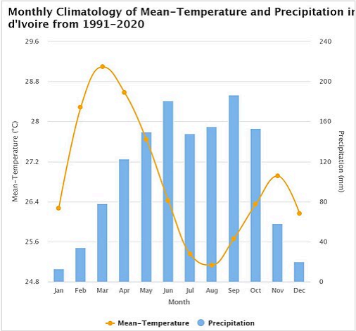
Climatologie mensuelle des températures moyennes et des précipitations en Côte d'Ivoire de 1991 à 2020 12 .
