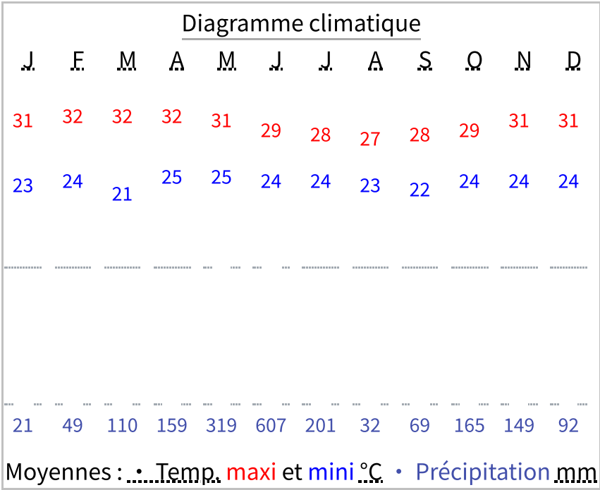
Relevé météorologique de Bouaké (Centre)
