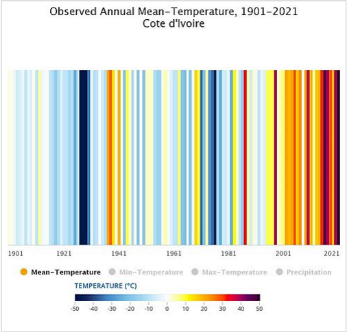
Température moyenne annuelle observée en Côte d'Ivoire de 1901 à 2021 12 .
