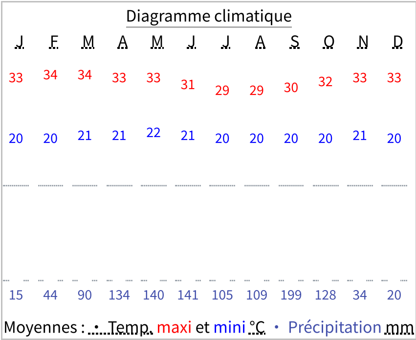
Relevé météorologique d'Odienné (Nord-ouest)
